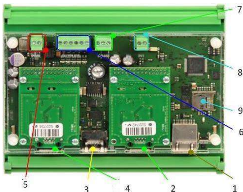
Рисунок 1. Внешний вид и расположение коммутационных элементов модуля ЦП
