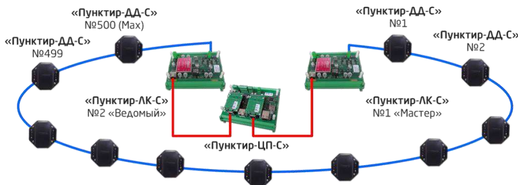
Рисунок 11. Кольцевая топология типа «кольцо» для периметра до 1,5 км.
