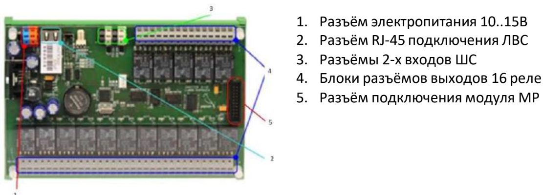
Рисунок 7. Внешний вид и расположение коммутационных элементов.
