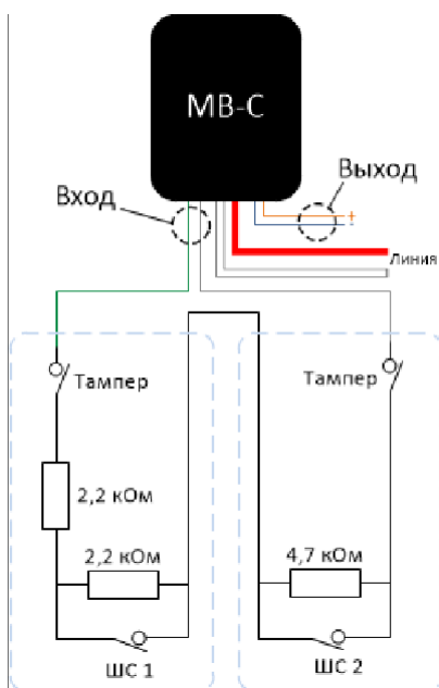
Рисунок 6. Схема подключения двух ШС к МВ.
