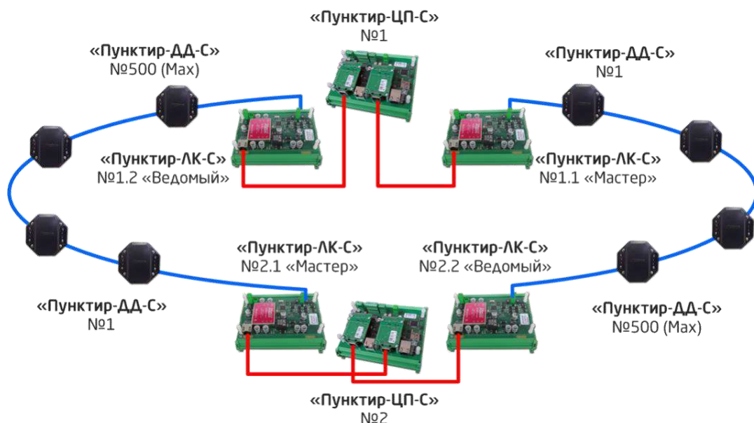
Рисунок 12. Кольцевая топология типа «Кольцо с резервированием»
