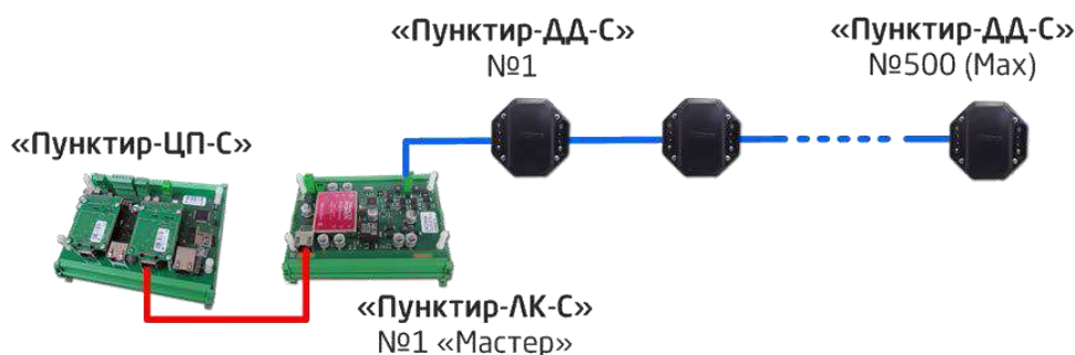
Рисунок 9. Линейная топология СОП («луч») с одним модулем ЛК.
