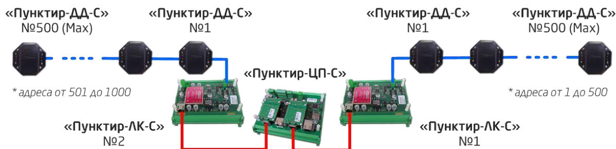
Рисунок 10. Линейная топология СОП («линия») с двумя модулями ЛК-С.
