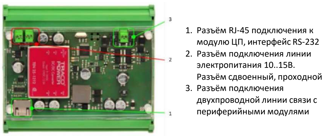
Рисунок 2. Внешний вид модуля ЛК и расположение коммутационных элементов
