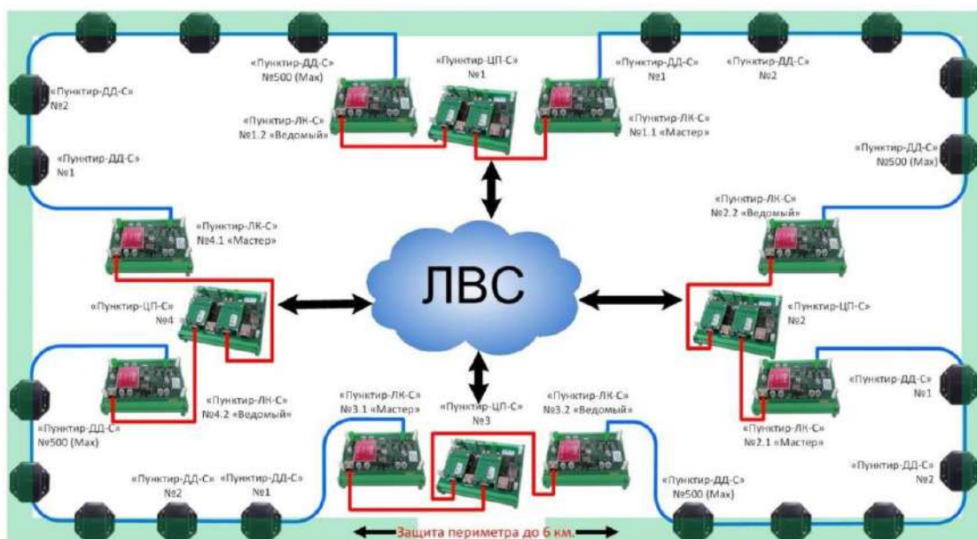
Рисунок 13. Обобщённая топология построения СОП.
